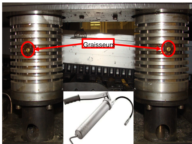
Lubrification de l'axe des turbines
