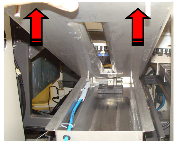
Démontage et nettoyage de la buse du fluxeur spray
